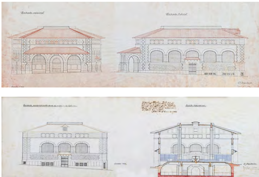
Figures 1 i 2: Proyecto de Mercado para la Ciudad de Felanitx . Façanes (principal i lateral) i Façana del carrer Alou i secció transversal. Aquest segon plànol conté anotacions que ens indiquen la data d'aprovació del projecte per part l'Ajuntament de Felanitx. Francesc Roca i Simó, 1931-1932. Font: Departament d'Urbanisme de l'Ajuntament de Felanitx
